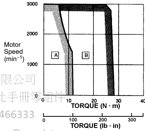
• SGMG-44A□A
