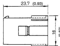
Cap: 172161-1 Socket: 170365-1
