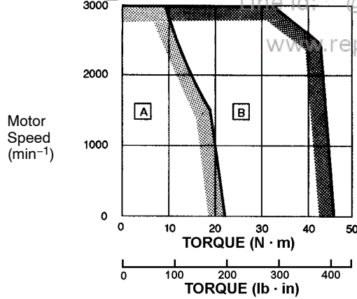
• SGMG-30A□A
