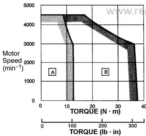
• SGMS-40A□A
