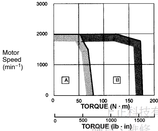
• SGMG-1AA□A
