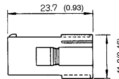
Cap: 172159-1 Socket: 170362-1 or 170366-1
