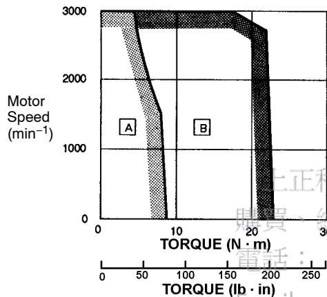
• SGMG-30A□A
