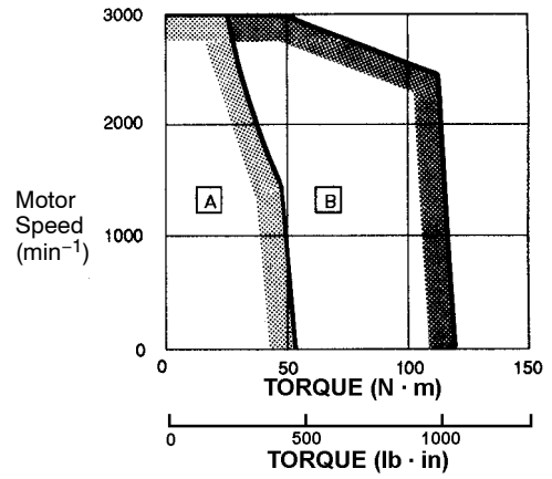
• SGMG-75A□A
