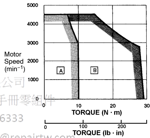
• SGMS-30A□A
