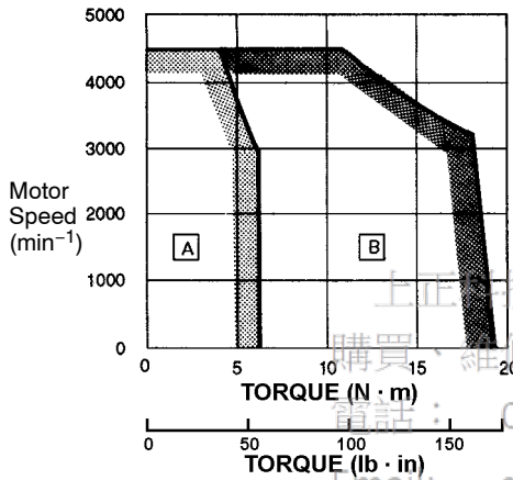
• SGMS-20A□A
