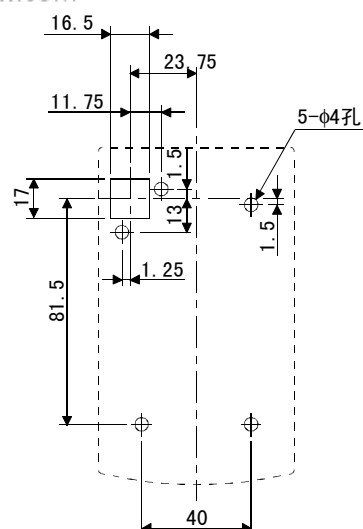
<面板开孔尺寸图>
